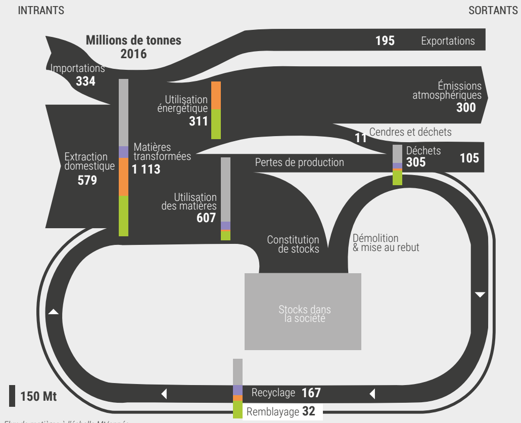
Figure 19. Circulation des matières dans l'économie française
