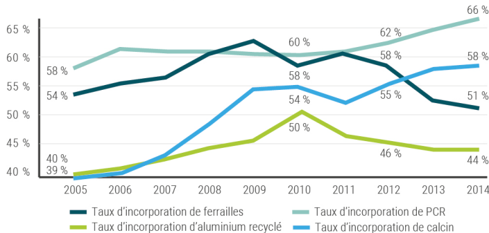
Figure 21. Évolution du taux d'incorporation de matières premières recyclables en France - 2005 à 2014
